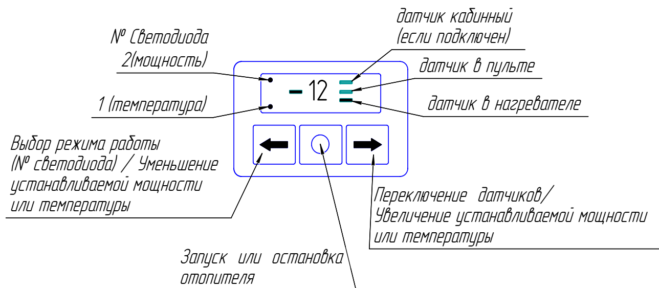
Рис. 6.1- Панель пульта
