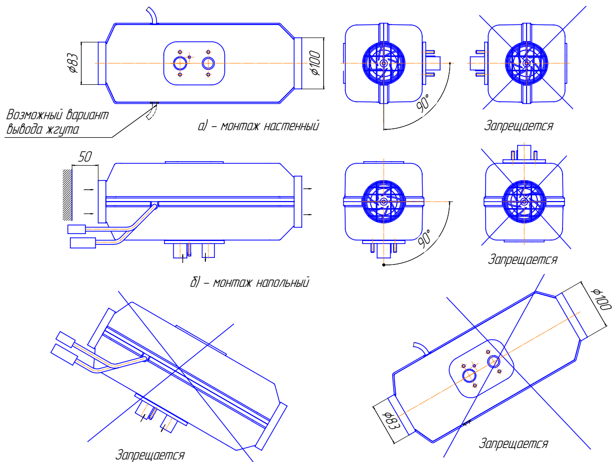
Рис. 7.1 – Варианты установки нагревателя
