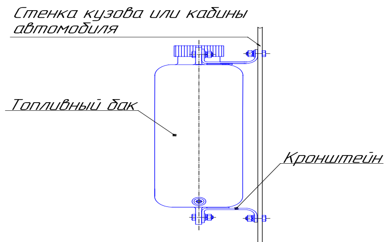
Рис. 7.5- Установка топливного бака на автомобиль.
