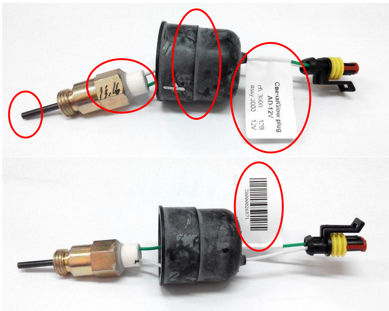
Оригинальная свеча Сб.3000 с элементом накаливания производства Япония
